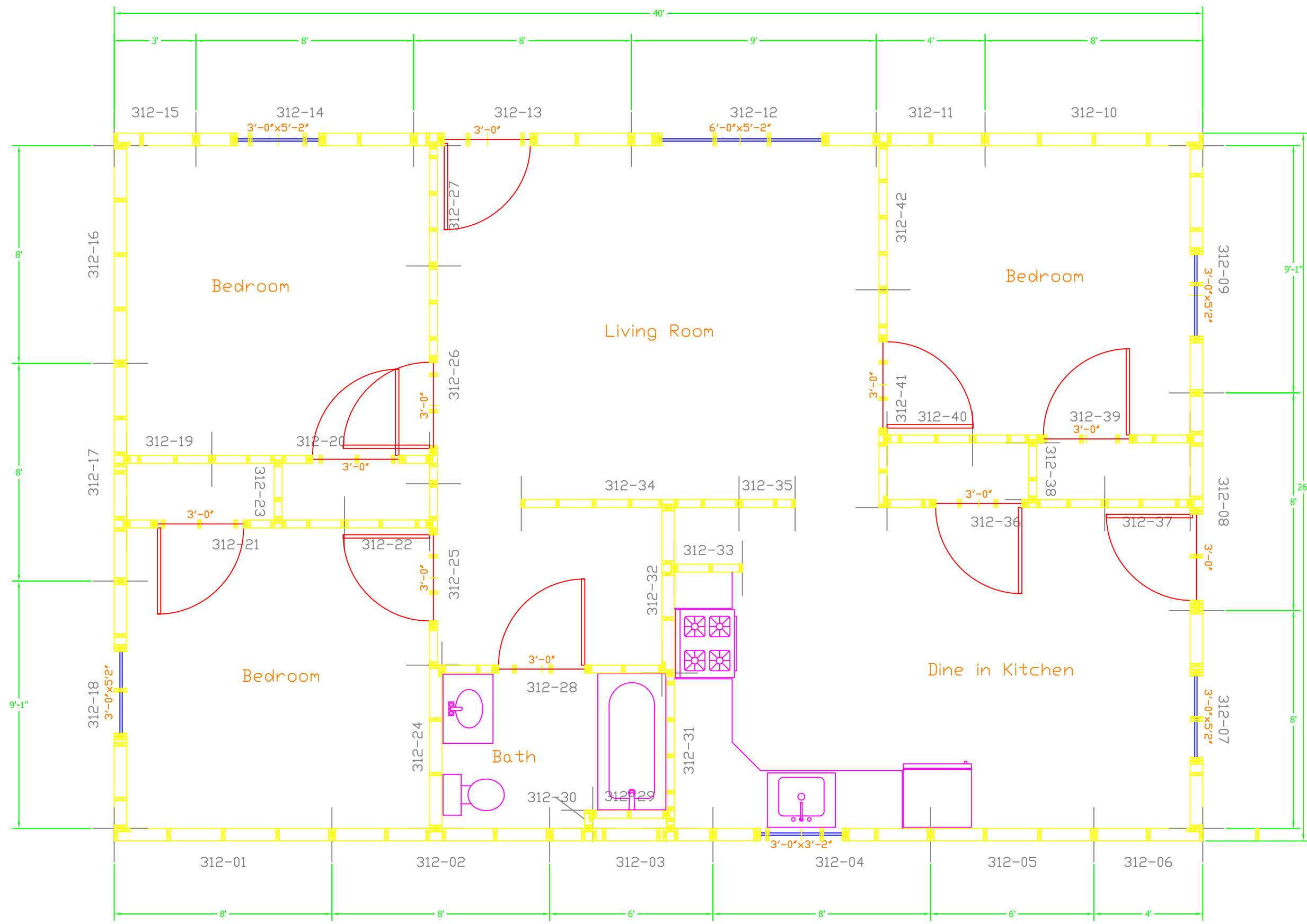
PLAN 312
